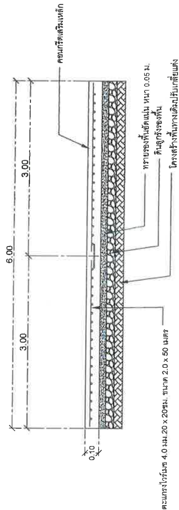
รูปตัดพื้นคอนกรีตเสริมเหล็ก GS
